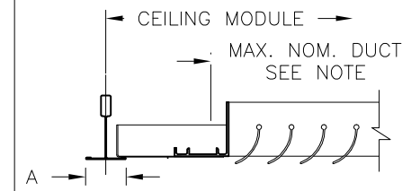
T-BAR LAY-IN PANELS: 3P 3PA A = 1\"/>
